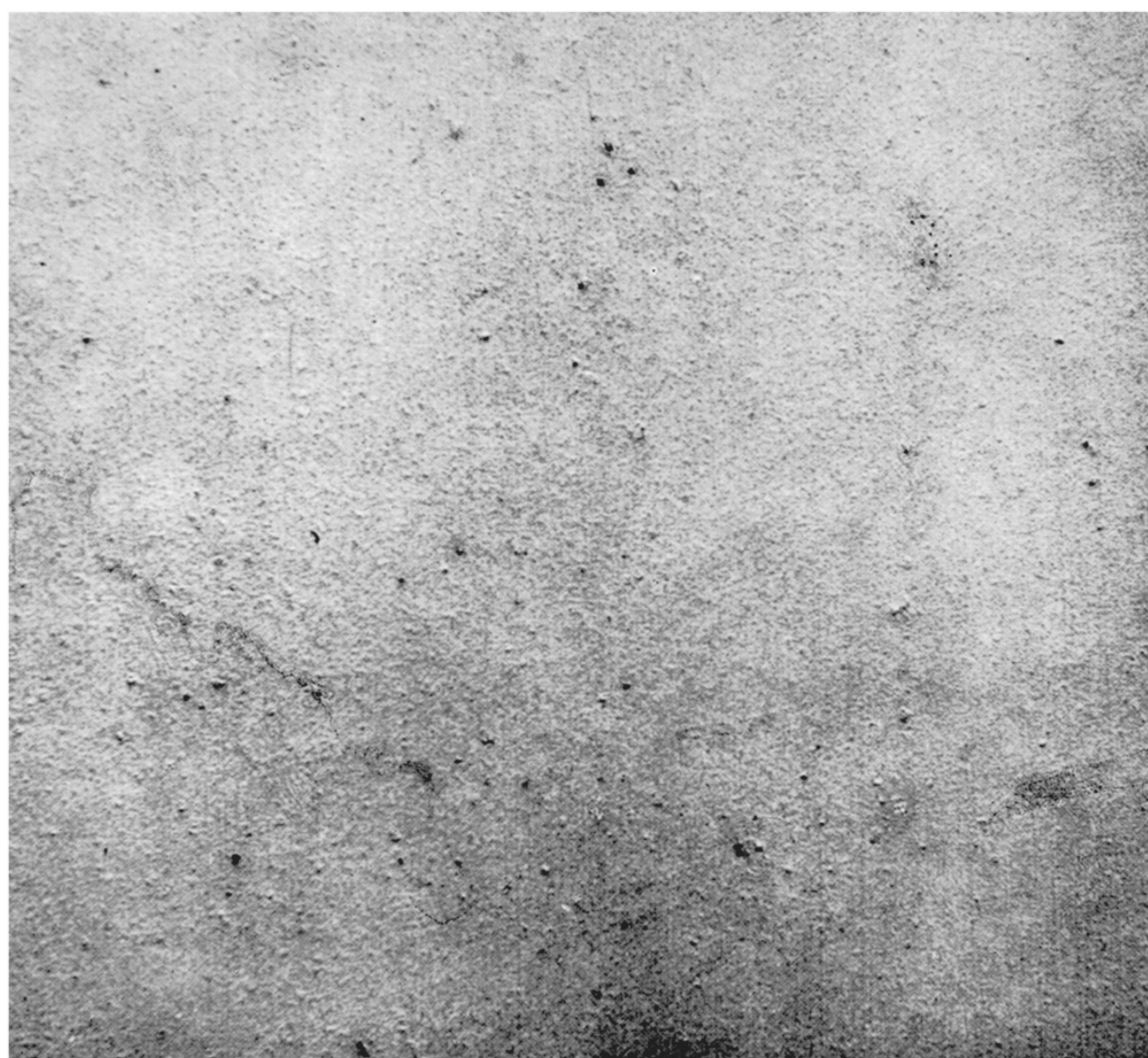
Рисунок 9 — Коррозия металла балл K1 (или Ri1 )
